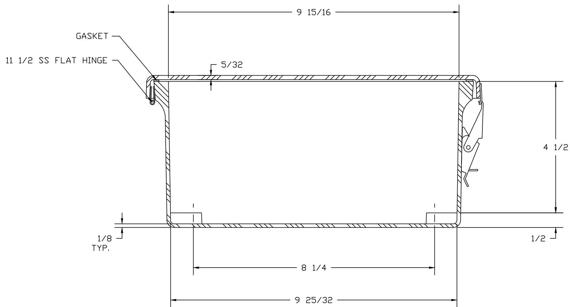
SECTION A-A
